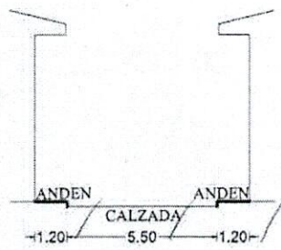
VIA VEHICULAR Escala: 1:200 CALLE 2 ENTRE CARRERA 11C Y CARRERA 12
