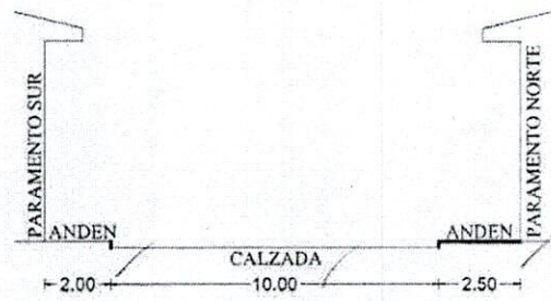
VIA VEHICULAR Escala: 1:200 CARRERA 11C ENTRE CALLE 2 Y CALLE 3
